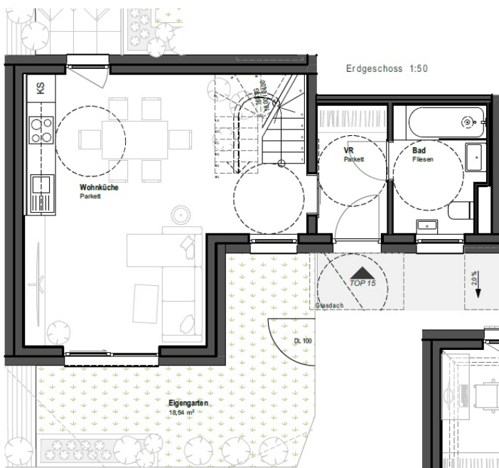
Überblick Erdgeschoss
