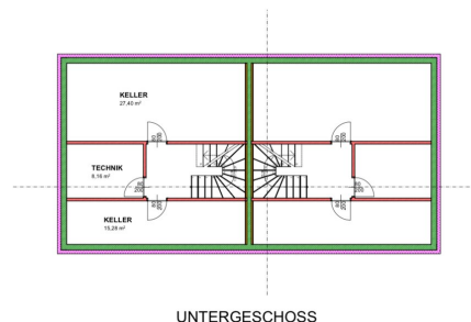
UNTERGESCHOSS
