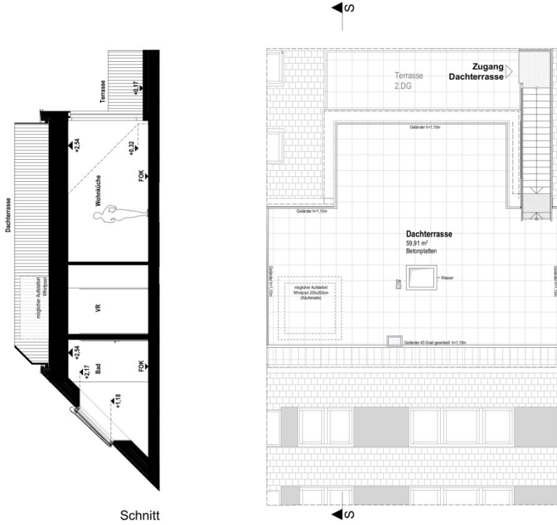
Schnitt
