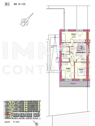
Grundrissplan | Top 6 Obergeschoss
