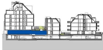
Schnitt
