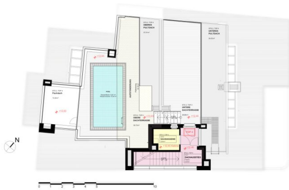
GRUNDRISS DG 1:100 TOP 4
