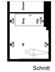
Schnitt
