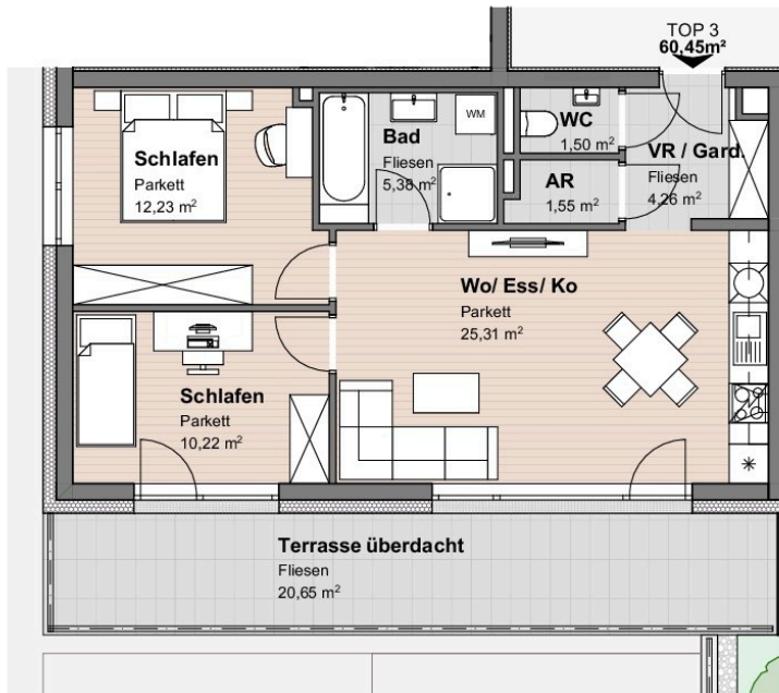
GRUNDRISS M=1:100
