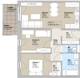
2. Obergeschoß M: 1: 100
