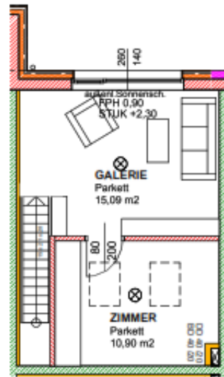
1. OBERGESCHOSS
