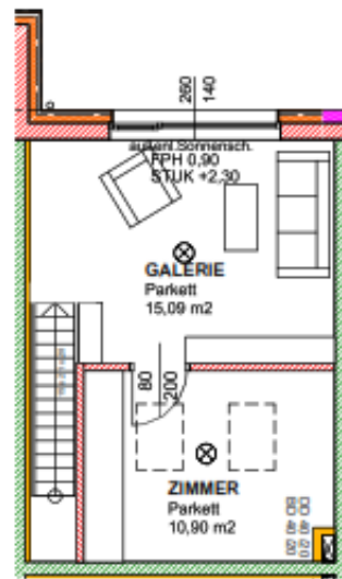
1. OBERGESCHOSS
