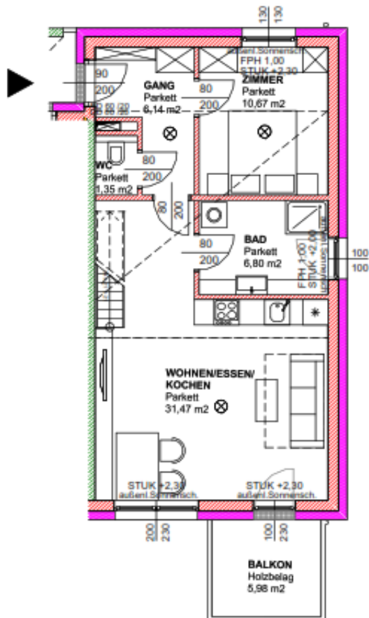
1. OBERGESCHOSS
