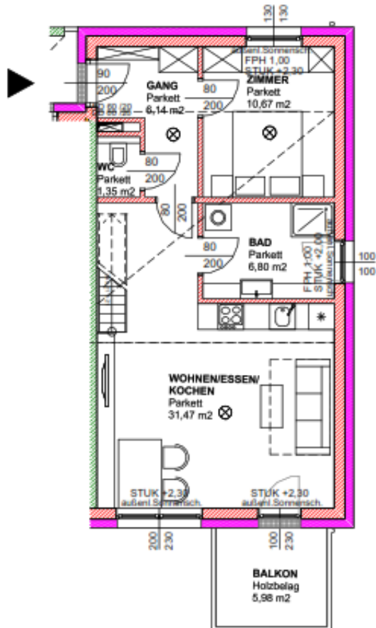
1. OBERGESCHOSS
