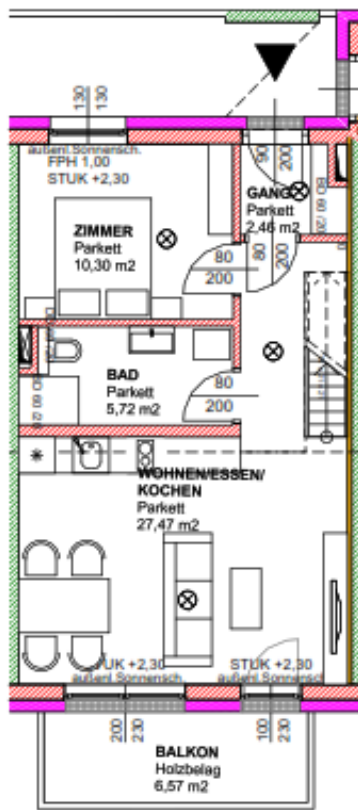
1. OBERGESCHOSS
