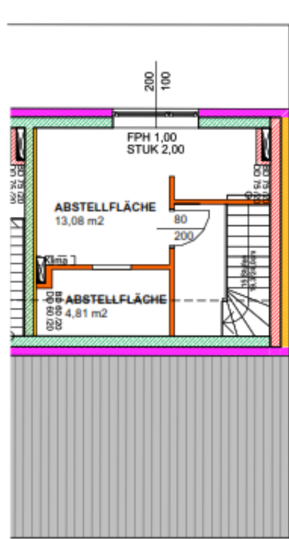
DACHBODEN
