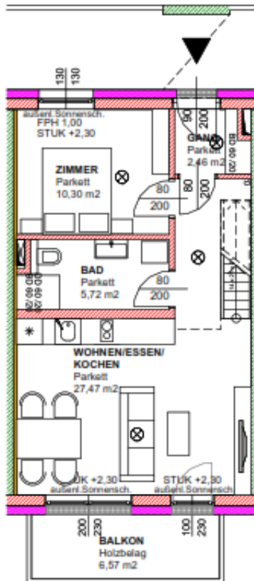
1. OBERGESCHOSS
