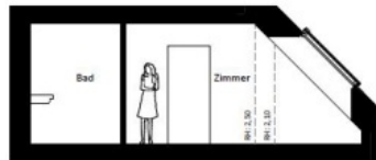
SCHNITT TOP 14
