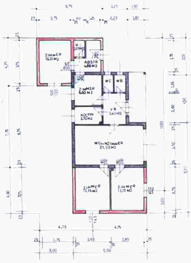
ERDGESCHOSS M=1:100
