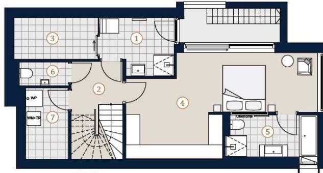
Untergeschoß
