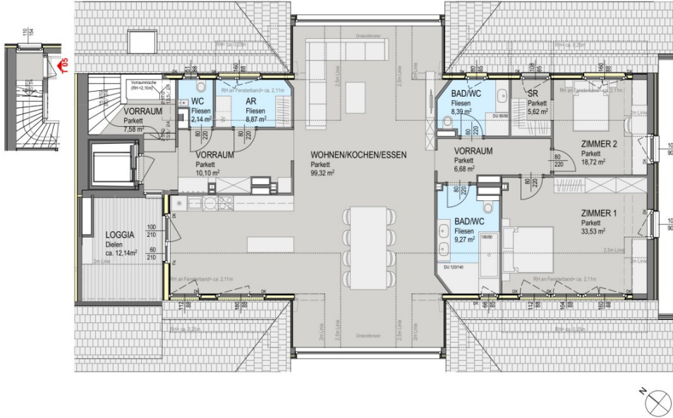
Grundriss Dachgeschoss
