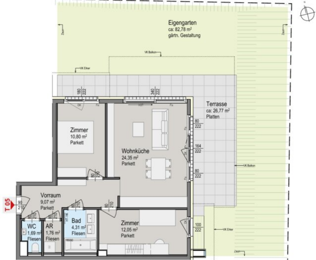
Grundriss Erdgeschoß
