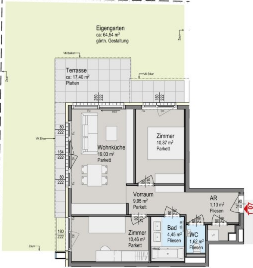
Grundriss Erdgeschoß
