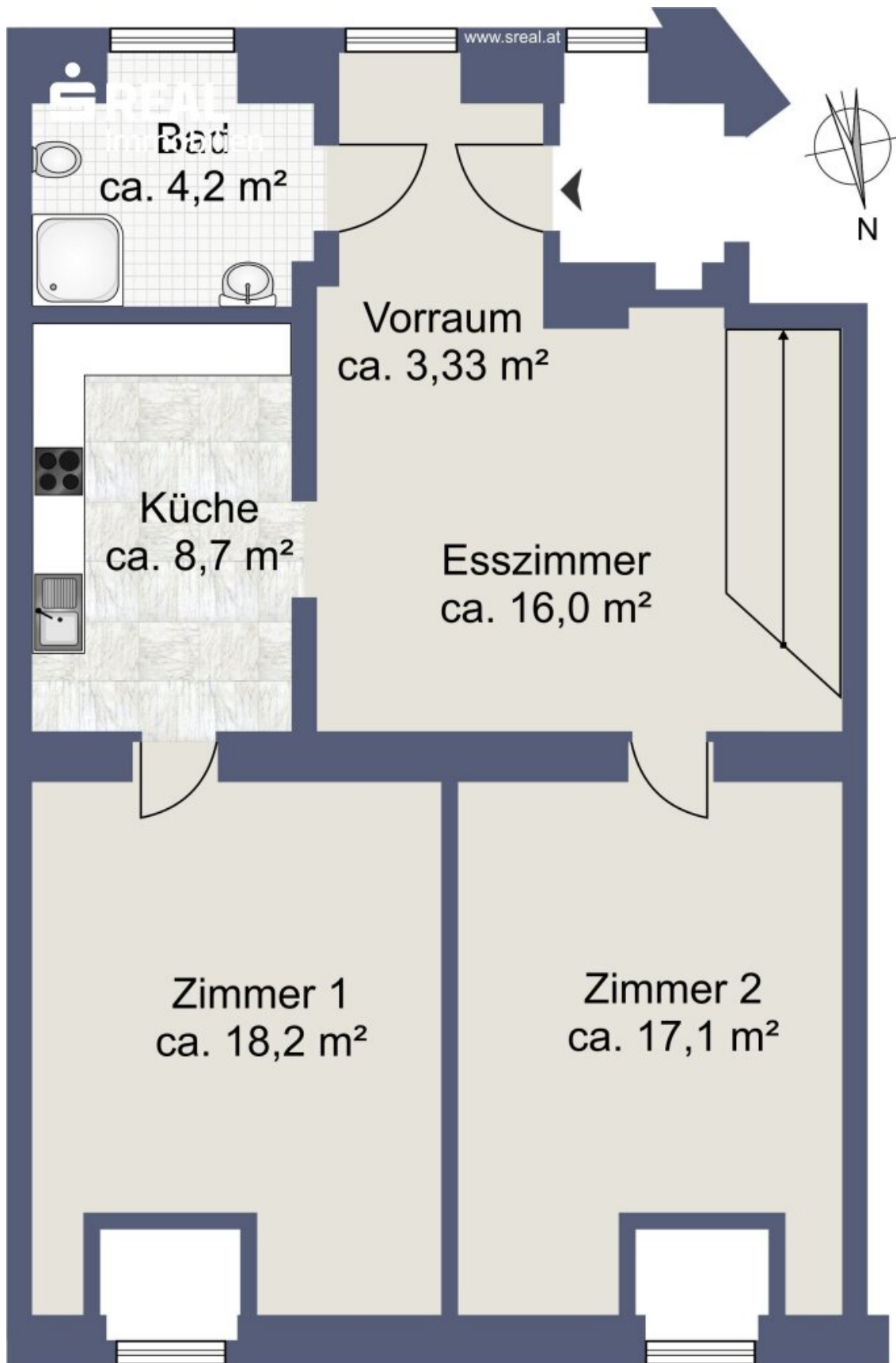
Skizze Erdgeschoss
