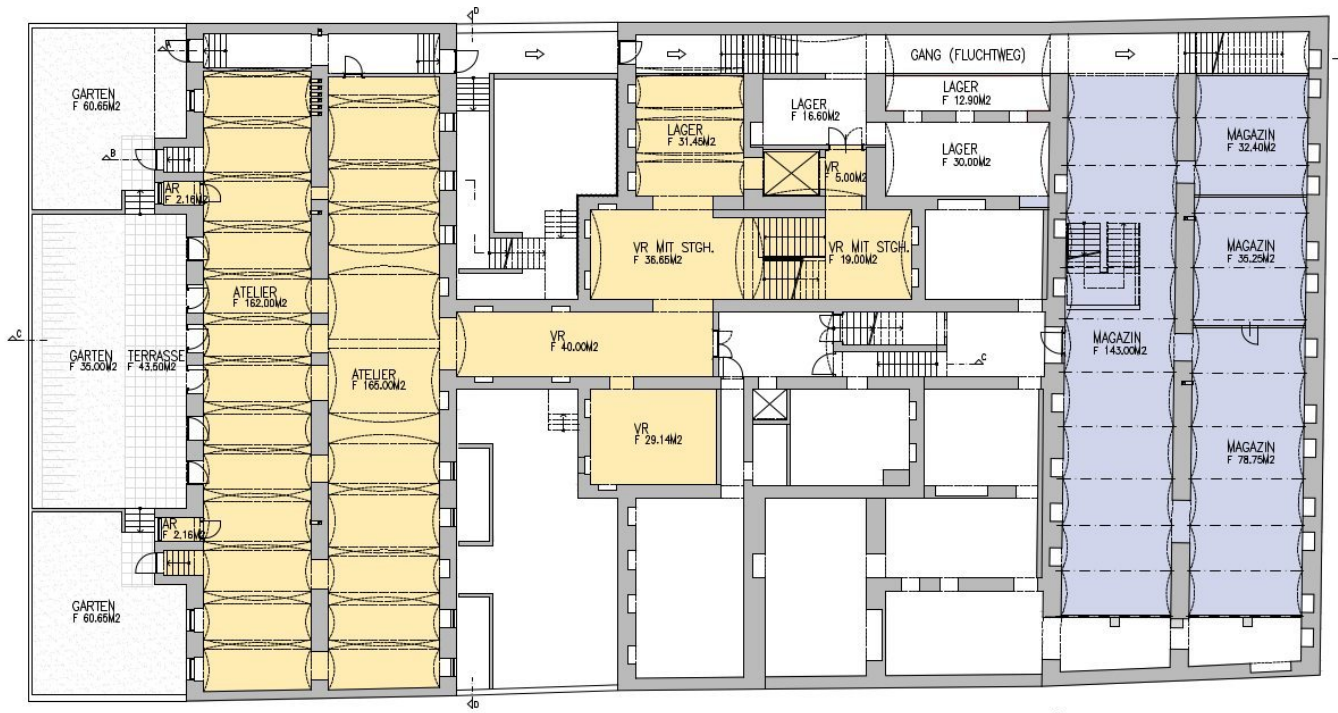
GRUNDRISS SOUTERRAIN
