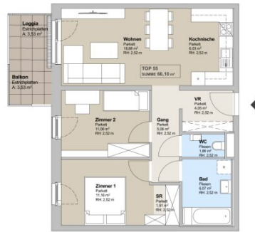
3. Obergeschoß M: 1: 100
