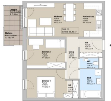
3. Obergeschoß M: 1: 100
