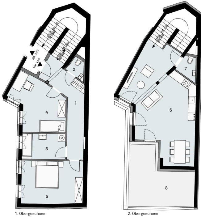
1. Obergeschoss
