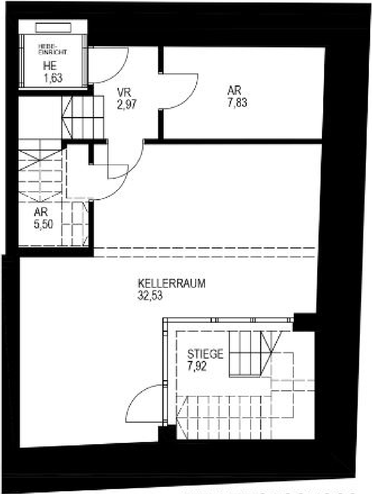
KELLERGESCHOSS
