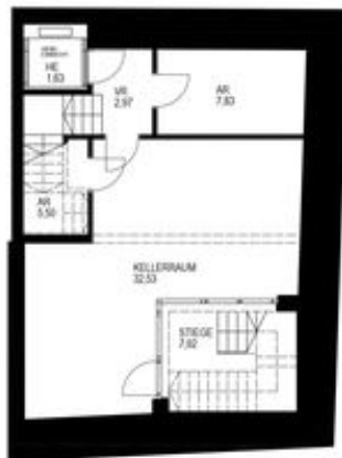
KELLERGESCHOSS
