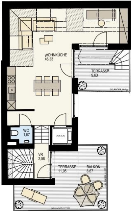
2. OBERGESCHOSS
