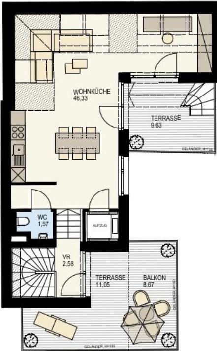
2. OBERGESCHOSS
