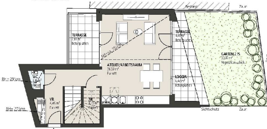
ERDGESCHOSS
