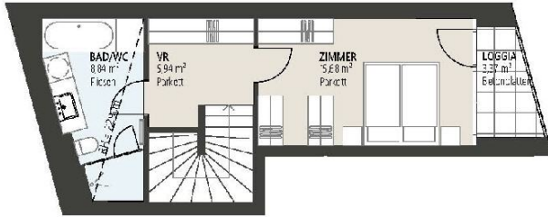
1.OBERGESCHOSS
