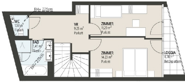
1. OBERGESCHOSS
