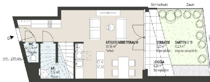
ERDGESCHOSS
