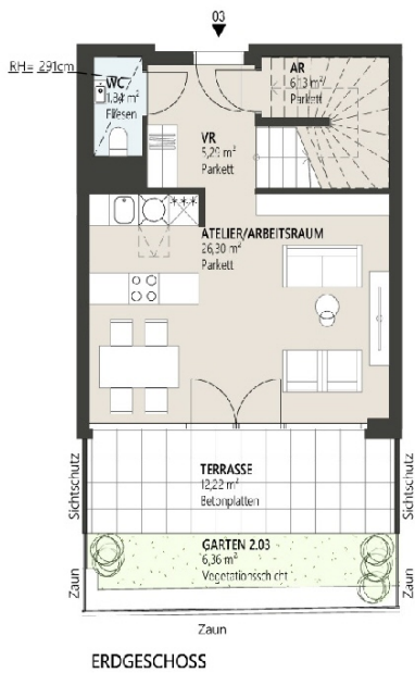
ERDGESCHOSS
