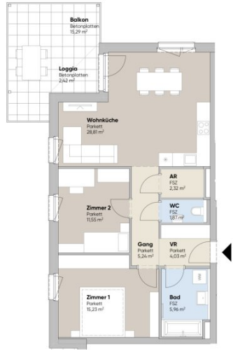
1. Obergeschoss
