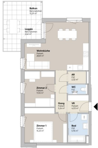
1. Obergeschoß
