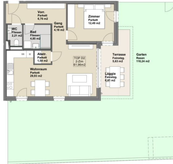
Top D 2 61,96 m 2
