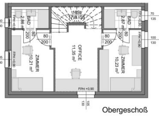
Obergeschoss
