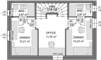
Obergeschoß
