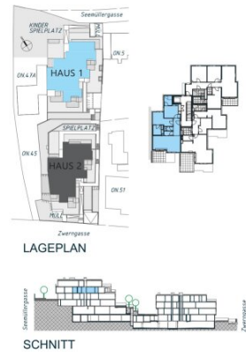
SCHNITT
