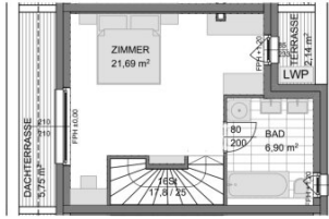
Dachgeschoß
