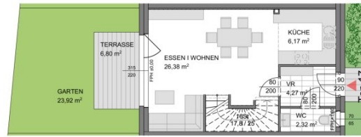
Erdgeschoß
