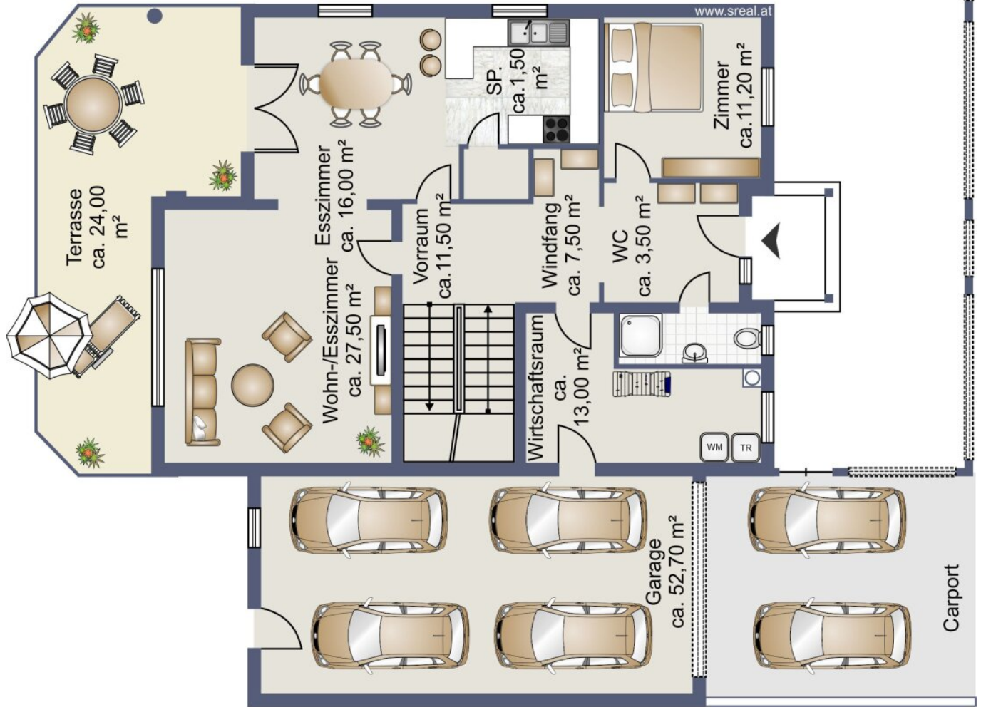
Skizze Erdgeschoss
