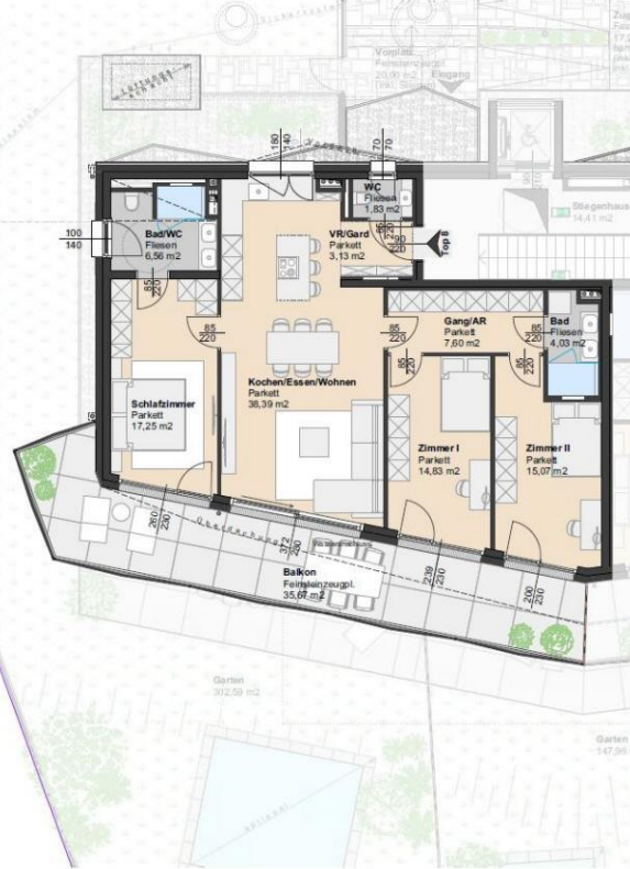
GRUNDRISS M= 1:250
