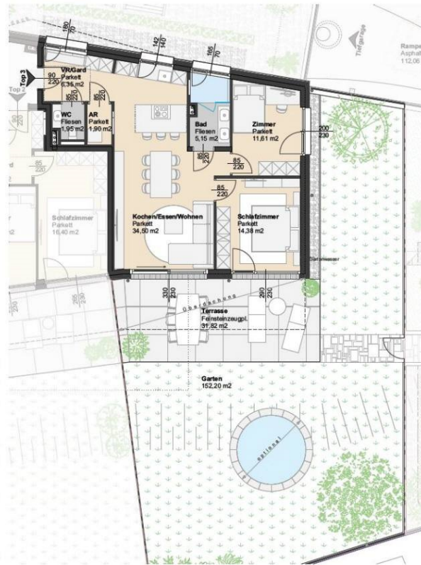
GRUNDRISS M= 1:250
