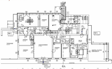
Einreichplan EG
