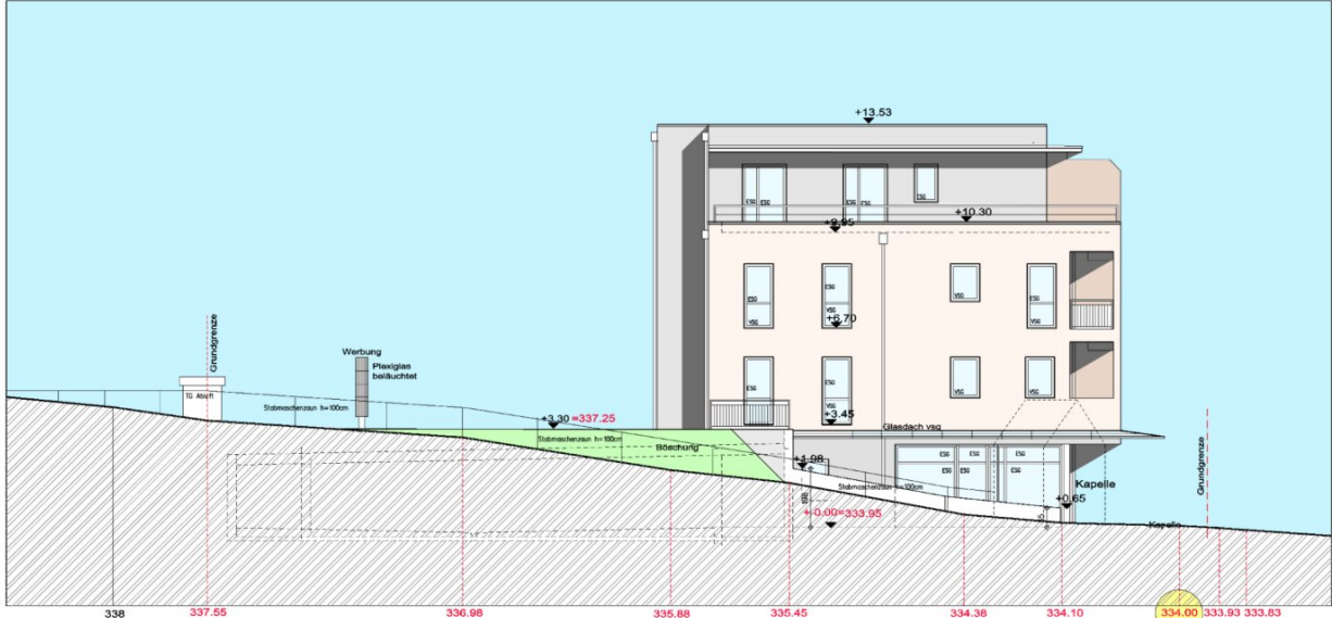
SÜDWESTANSICHT mit Strassenprofil = Naturaufnahme
