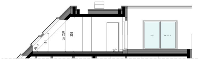
Schnitt 43.C
