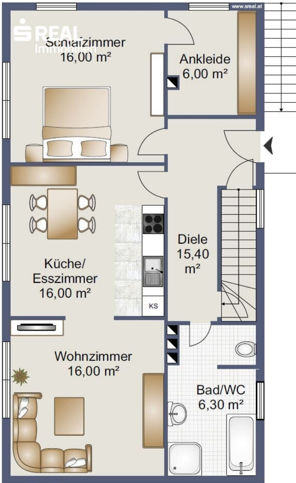
Skizze Erdgeschoss
