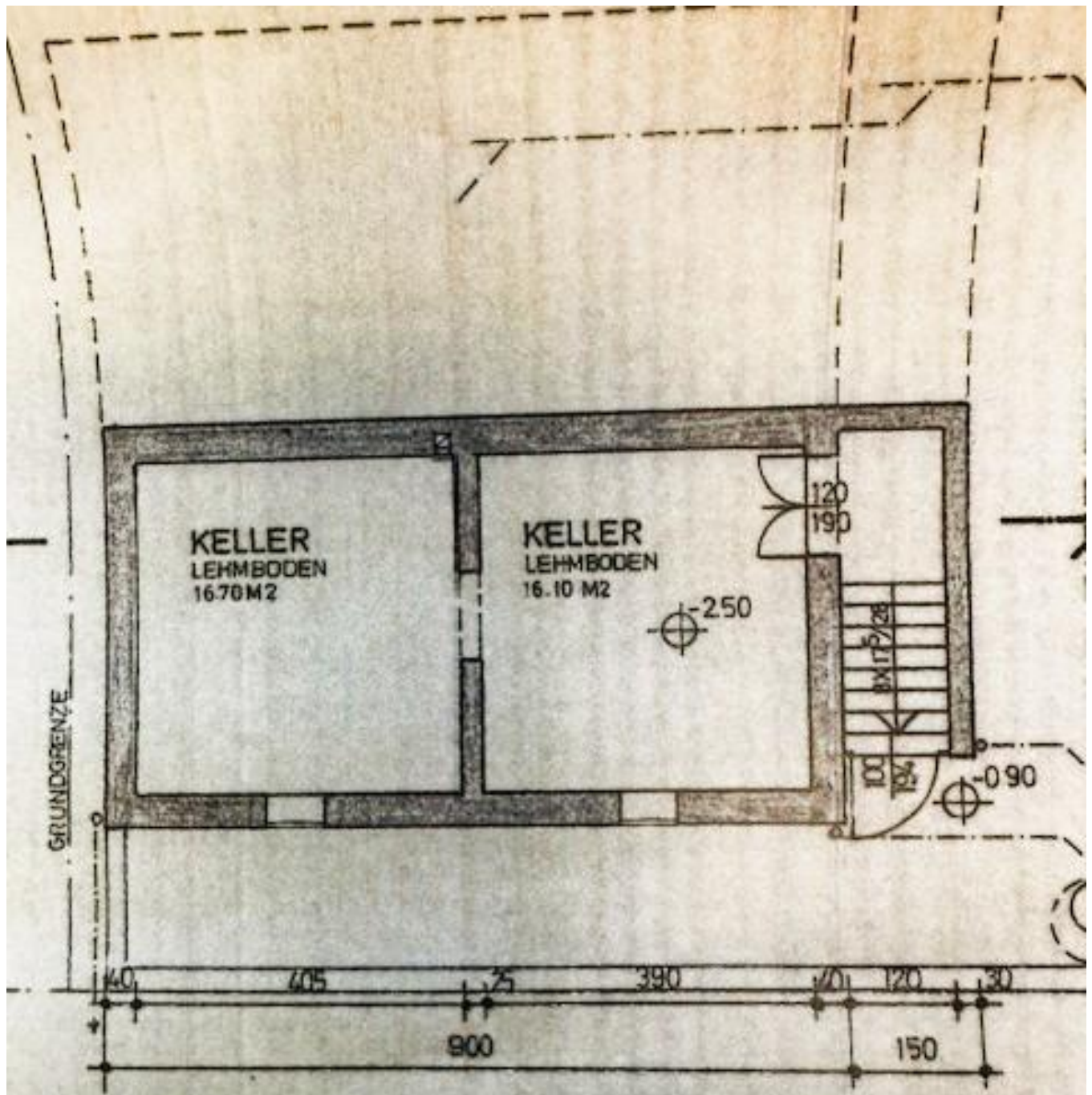
GRUNDRISS KELLER
