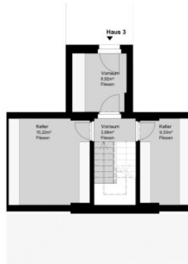
HAUS 3 - KELLERGESCHOSS / TIEFGARAGE
