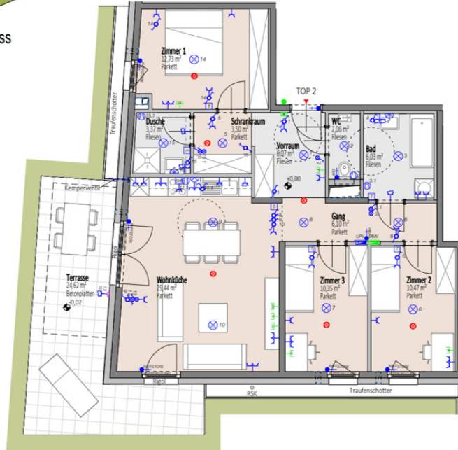
Grundriss mit Möblierungsvorschlag - Möbel nicht enthalten
