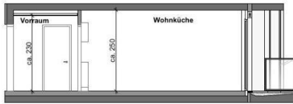
Schnitt | M 1:100
