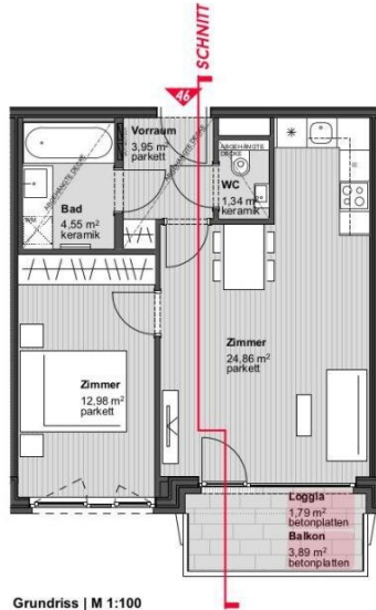
Grundriss | M 1:100
