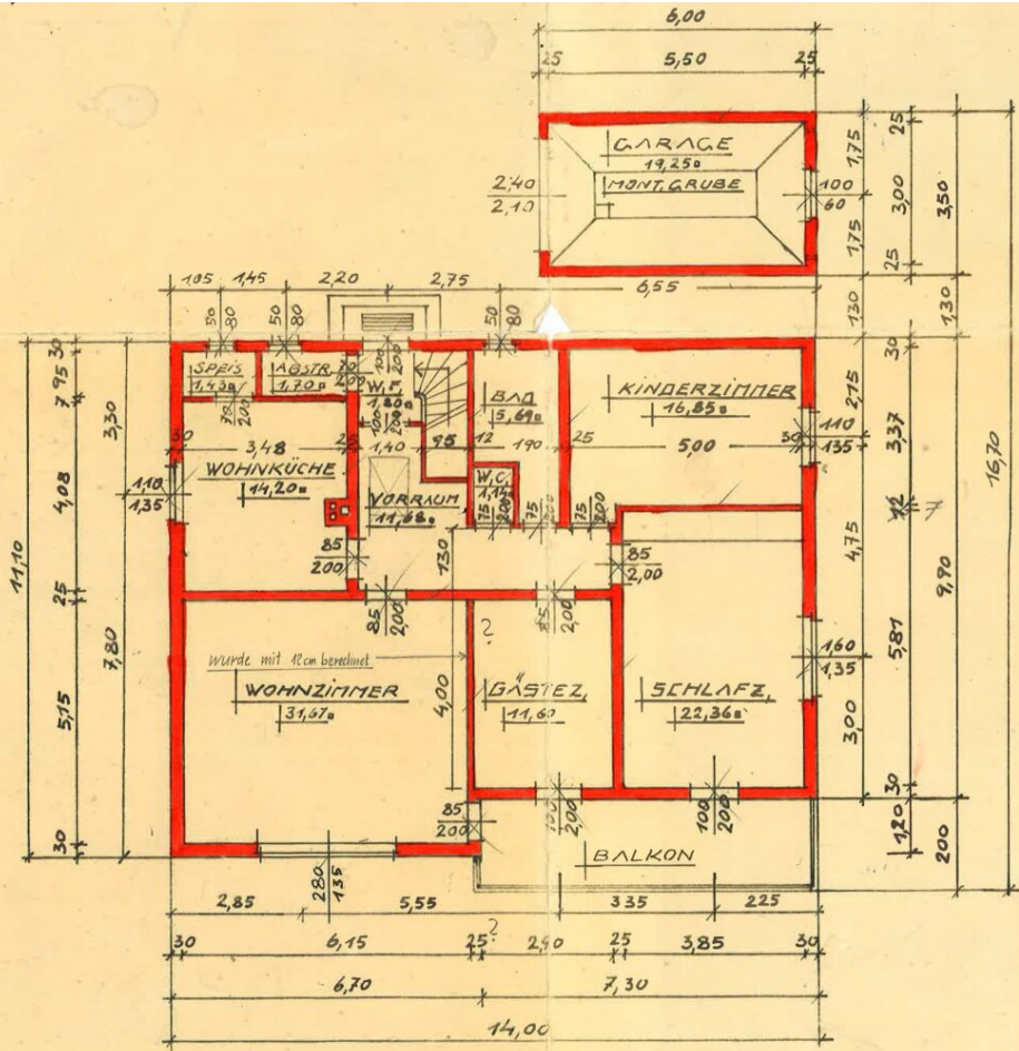
ERDGESCHOSS T + V + BALKON
