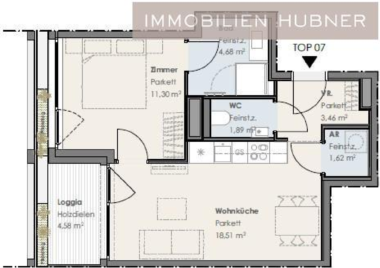
GRUNDRISS TOP 07
