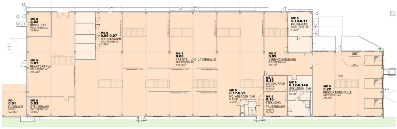
ERDGESCHOSS | MIETENEHIT 9 | M=1:250 | GESAMTFLÄCHE : 2164,24 m 2
