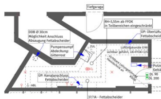
Untergeschoss Haustechnik Gastro 1:100
